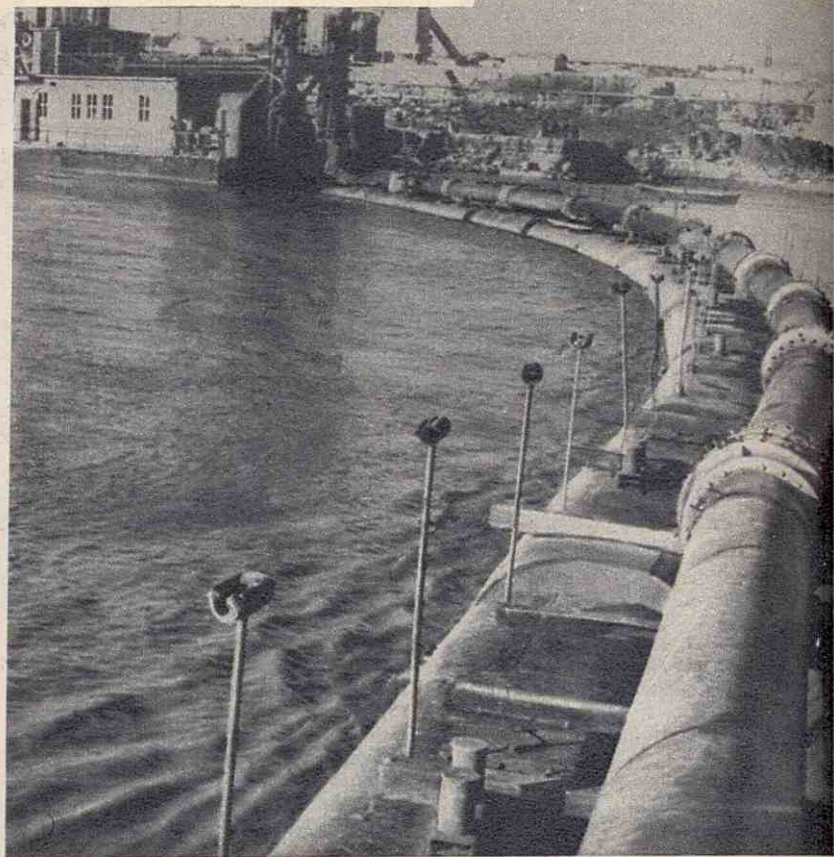
↑ Молдавская ССР. На строительстве Дубоссарской ГЭС закончено сооружение плотины и затопление котлована. На снимке: земснаряд размывает перемычку для пропуска днестровской воды.
